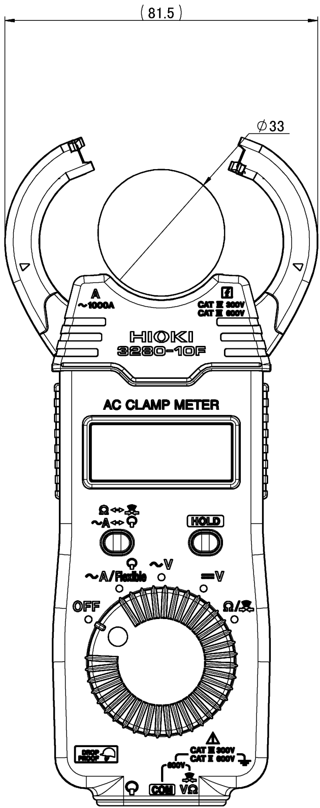
ジョーを開いた図
